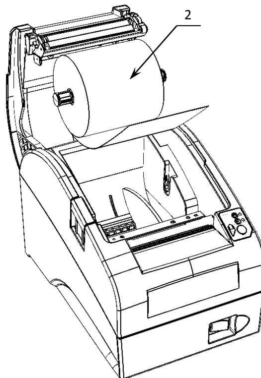
Рисунок 12. Установка ЧЛ
